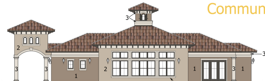
Right Elevation
